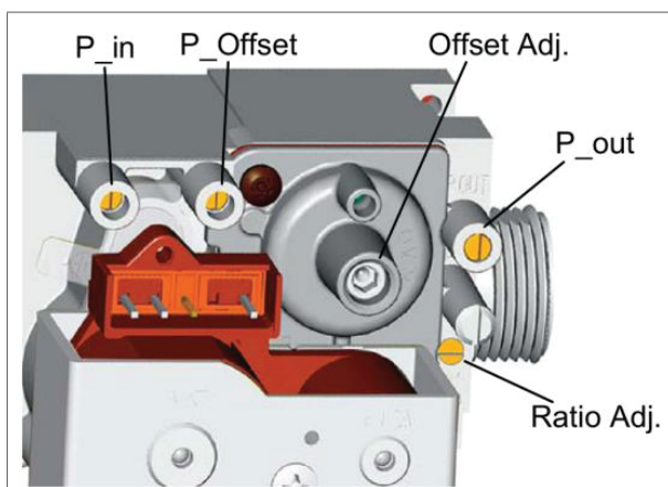
Figure 23 - Composants majeurs de la vanne de gaz
