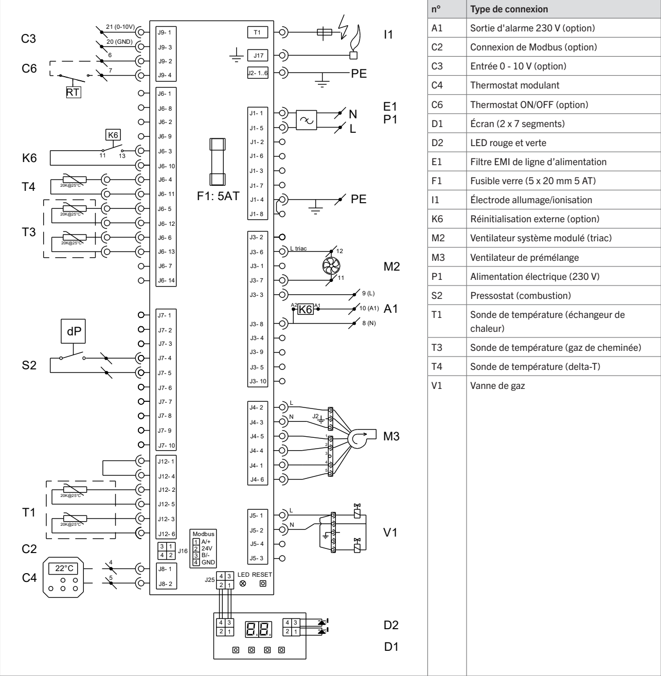
Figure 26 - Schéma de câblage AC
