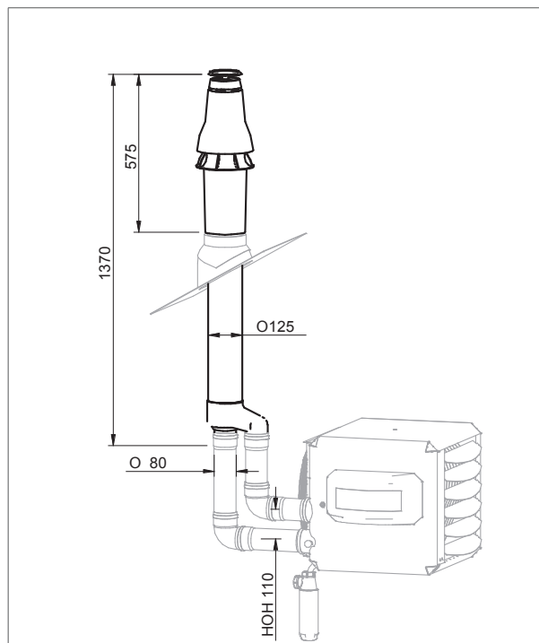
Figure 15 - Terminal vertical des gaz de cheminée HR10 - HR60
