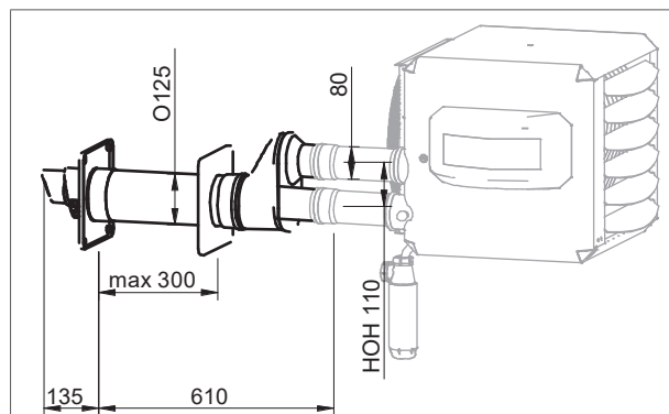
Figure 17 - Terminal horizontal des gaz de cheminée HR10 - HR60
