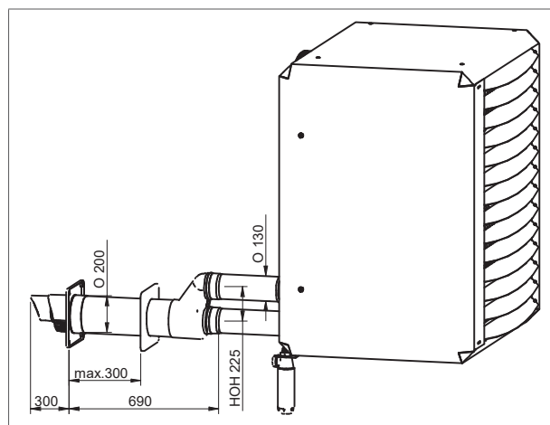
Figure 18 - Terminal horizontal des gaz de cheminée HR80 - HR120
