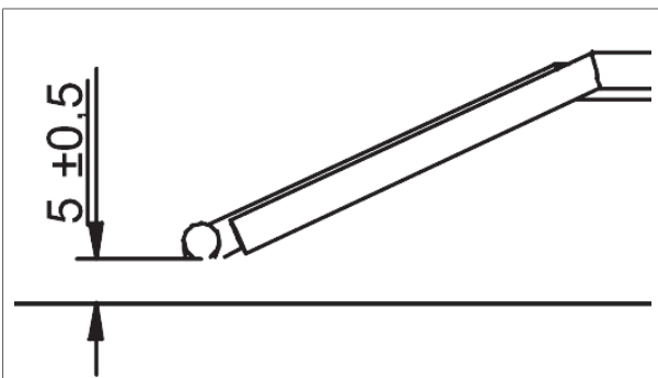
Figuur 24 - Afstand tussen de elektrode en de brander
