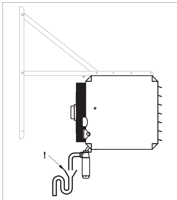
Figuur 19 - De condensafvoerleiding
