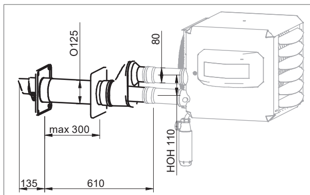
Figuur 17 - Horizontale uitmonding HR10 - HR60
