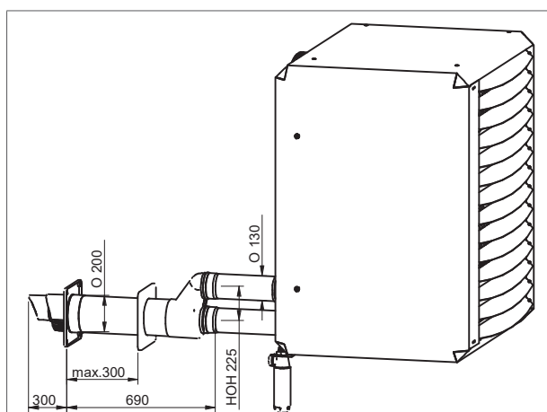
Figuur 18 - Horizontale uitmonding HR80 - HR120
