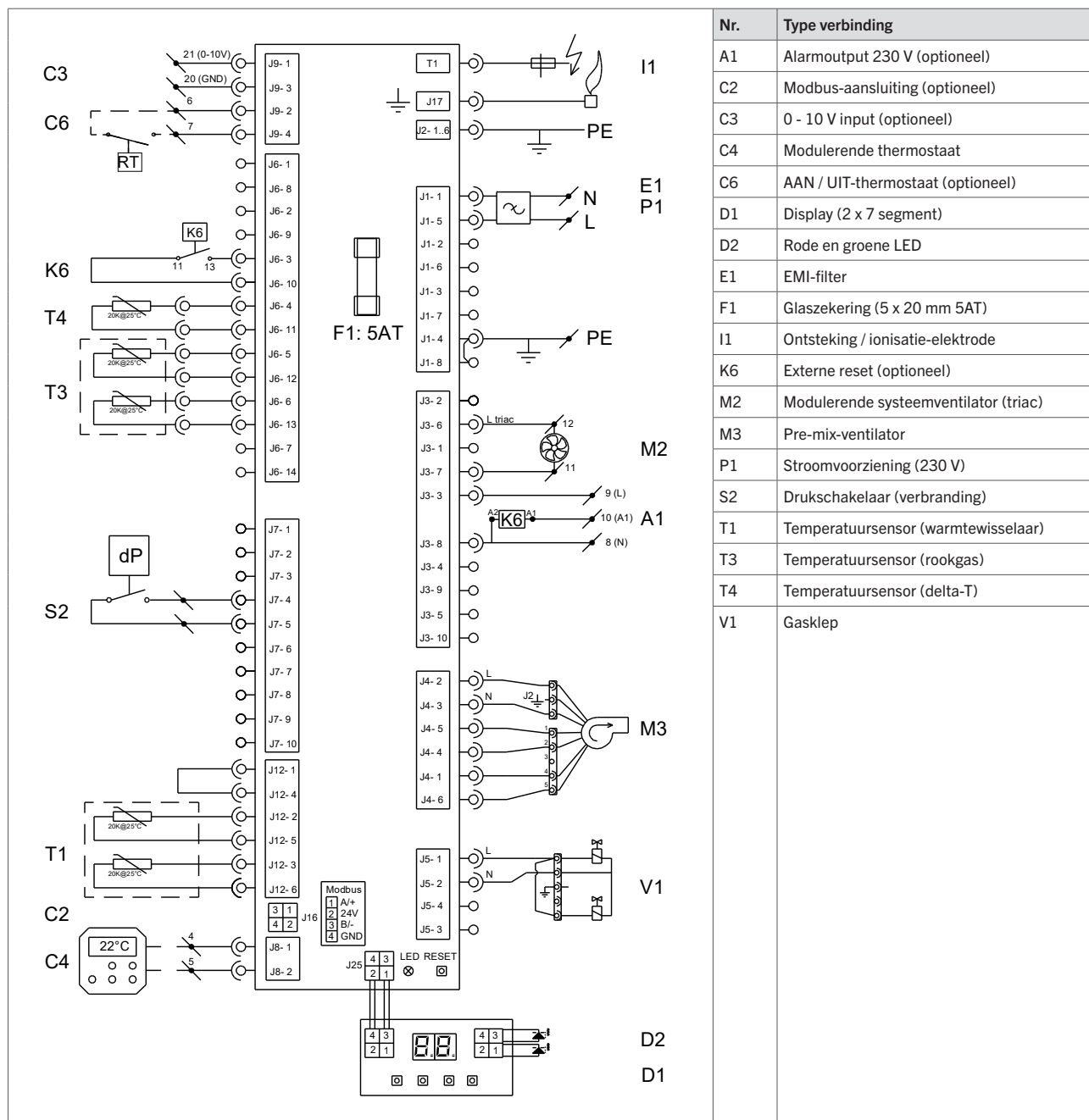
Figuur 26 - Elektrisch schema AC
