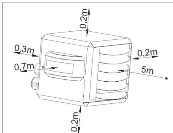
Figuur 5 - Minimale vrije ruimte rondom de luchtverwarmer
