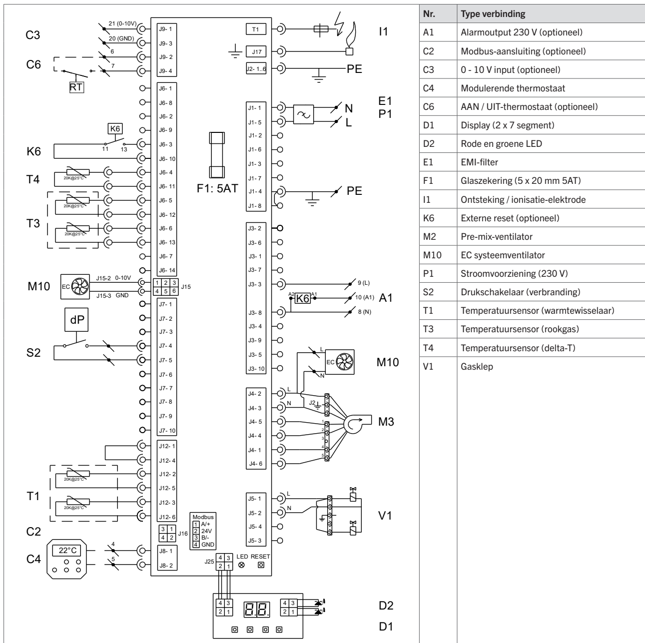
Figuur 28 - Elektrisch schema EC
